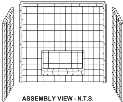
ASSEMBLY VIEW - N.T.S.
