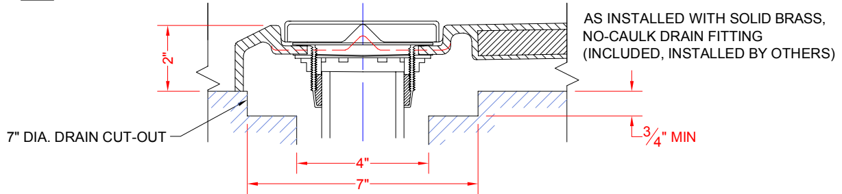
SECTION A-A - SCALE: 3" = 1'-0"
