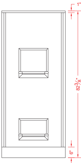
FRONT ELEVATION - SCALE: \frac{3}{8}'' = 1'-0''
