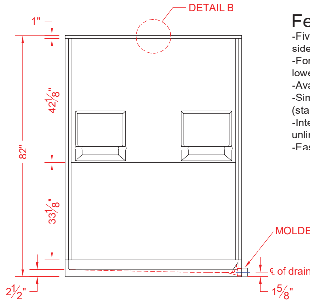
FRONT ELEVATION - SCALE: \frac{3}{8} " = 1'-0"
