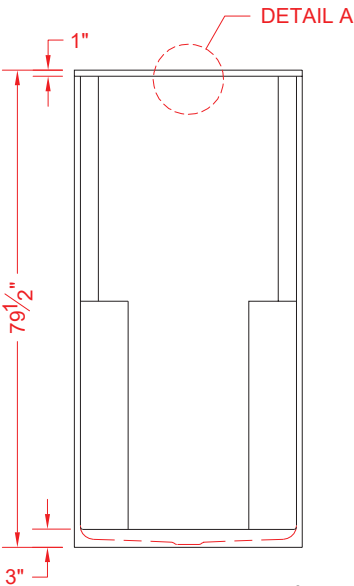
FRONT ELEVATION - SCALE: 3/8" = 1'-0"
