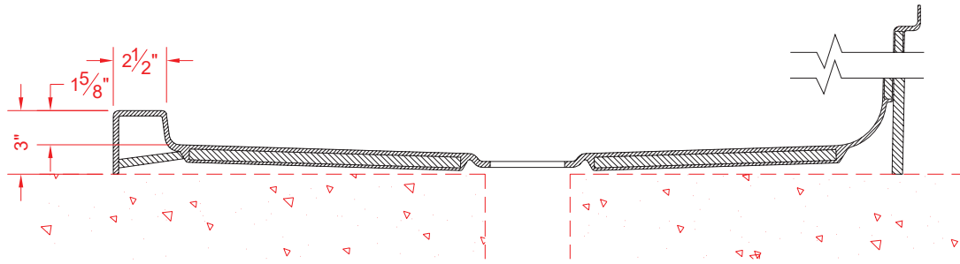
SECTION A-A Scale 1 : 8
