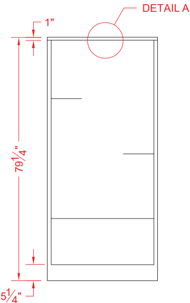
FRONT ELEVATION - SCALE: 3/8" = 1'-0"
